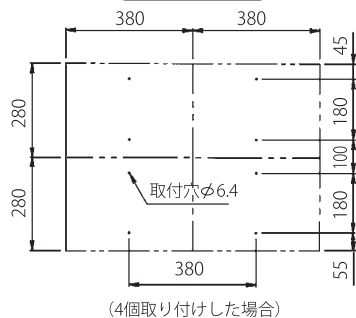
取付ピッチ図
