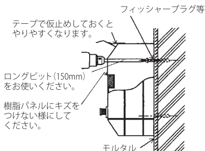
取付図例
