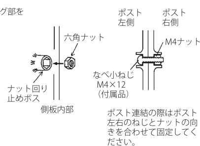
左右連結方法
