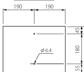
取付ピッチ図
